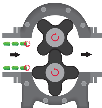
Běžná konstrukce čerpadla s rotačními písty
