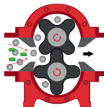
Čerpadlo s rotačními písty se systémem InjectionSystem
