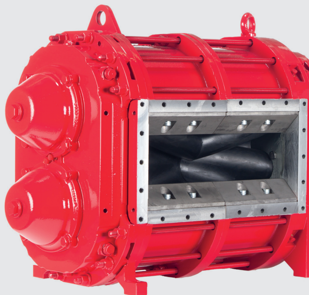
Čerpadlo s rotačními písty vybavené systémem InjectionSystem
